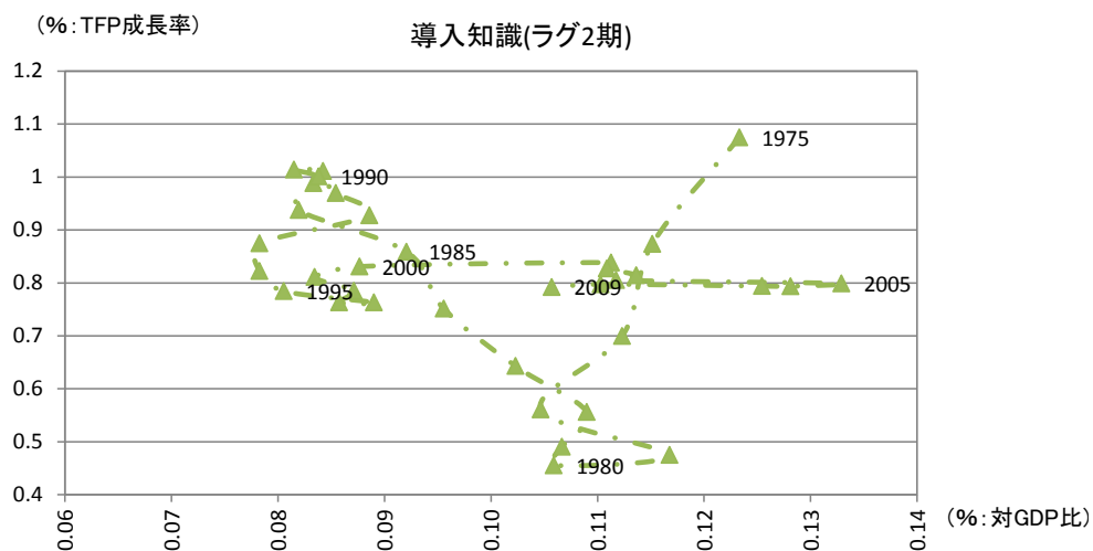
参考図表 A-9 TFP 成長率と研究集約度の分布(導入知識)
